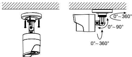
Рисунок 1. Установка камеры на потолок.
